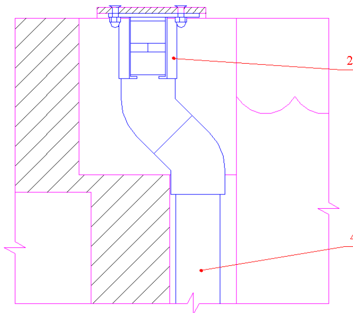
Рисунок 10 (скиммерной бассейн)
