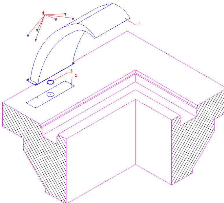
Рисунок 17 (переливной бассейн)
