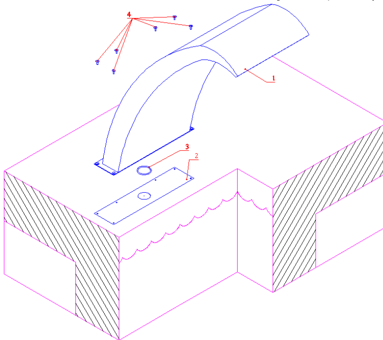
Рисунок 17 (переливной бассейн)
