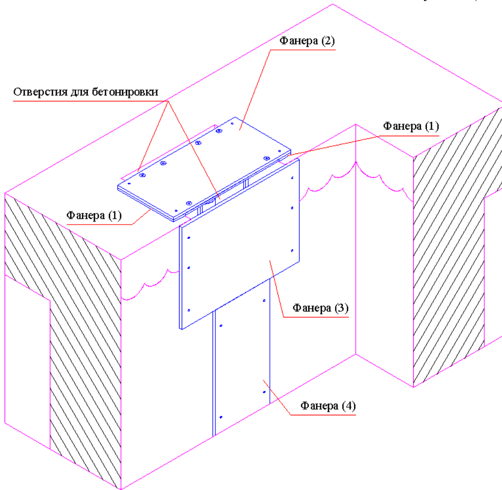
Рисунок 15 (переливной бассейн)
