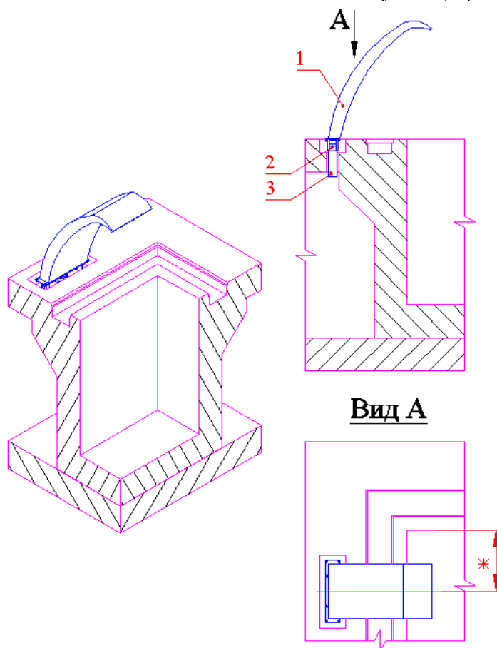
Рисунок 6 (переливной бассейн)
