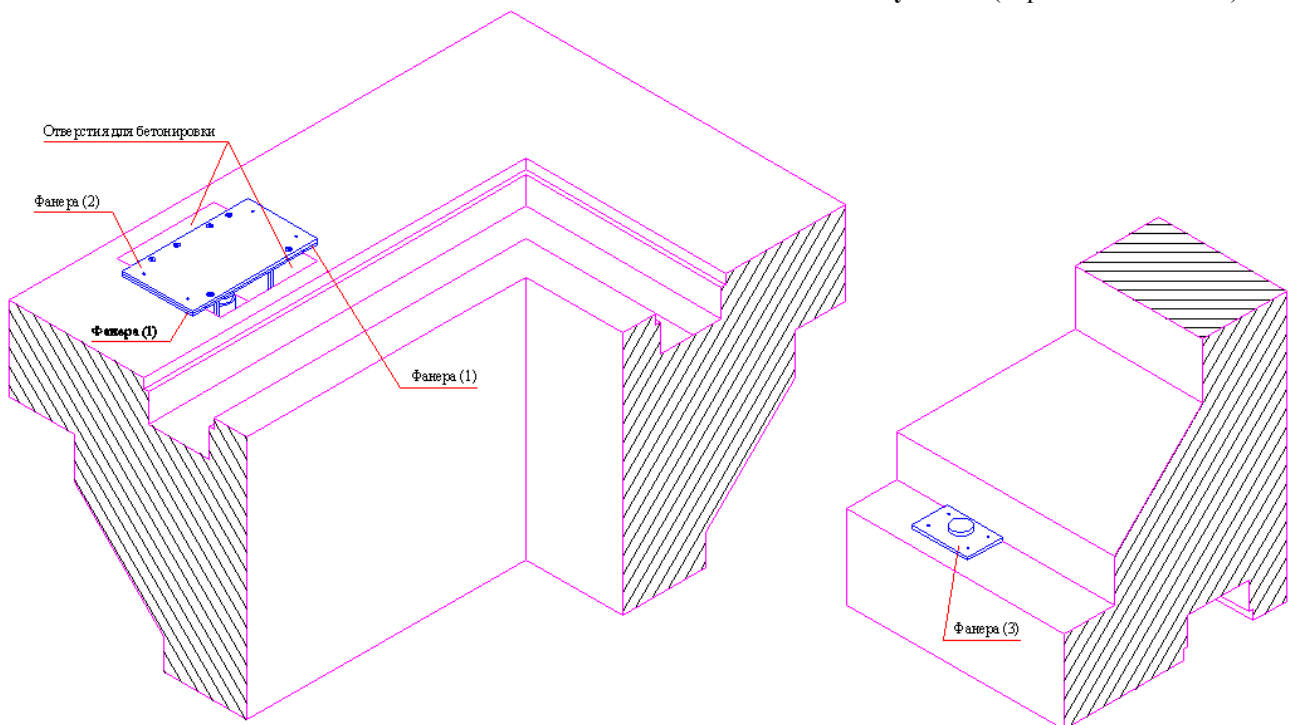
Рисунок 15 (переливной бассейн)
