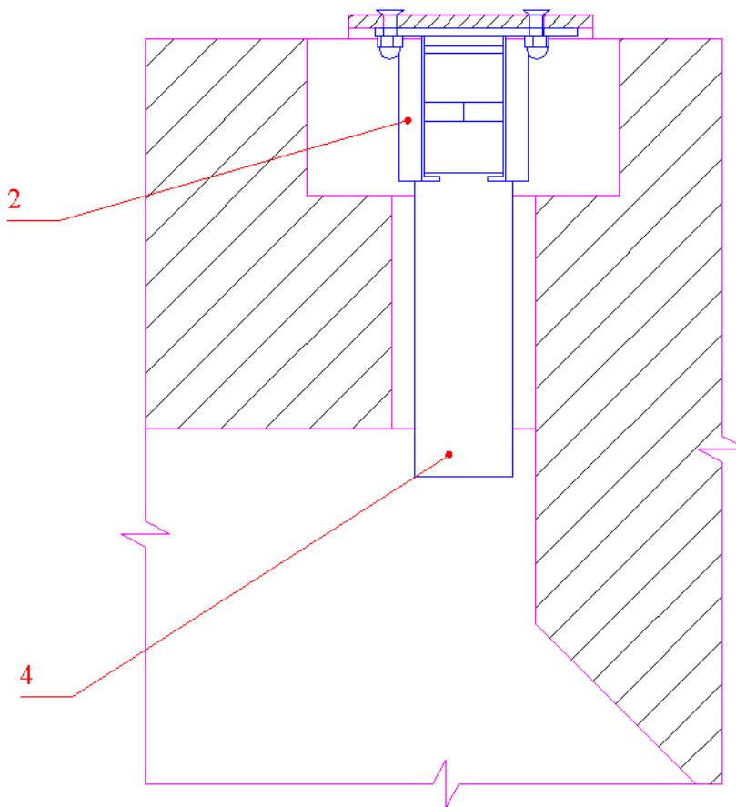
Рисунок 11 (переливной бассейн)
