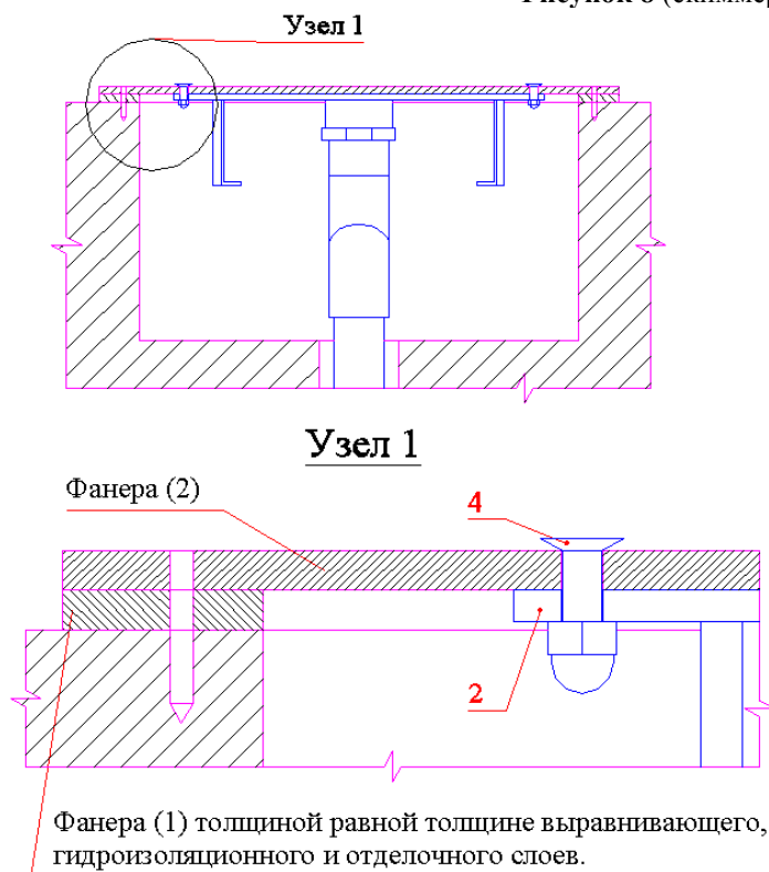
Рисунок 8 (скиммерной бассейн)
