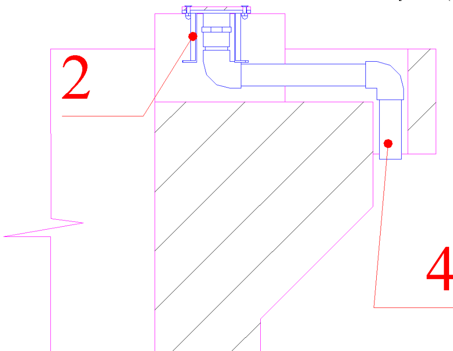
Рисунок 11 (переливной бассейн)
