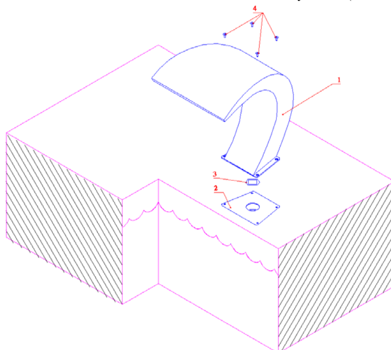
Рисунок 16 (скиммерной бассейн)
