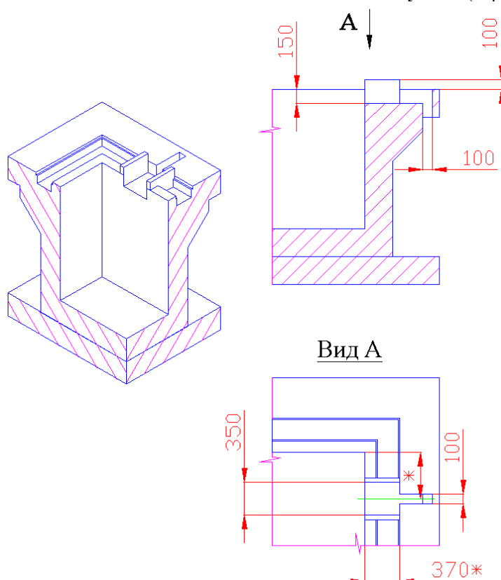
Рисунок 4 (переливной бассейн)
