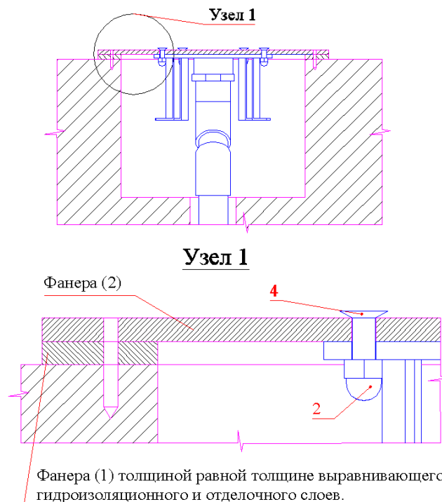
Рисунок 8 (скиммерной бассейн)
