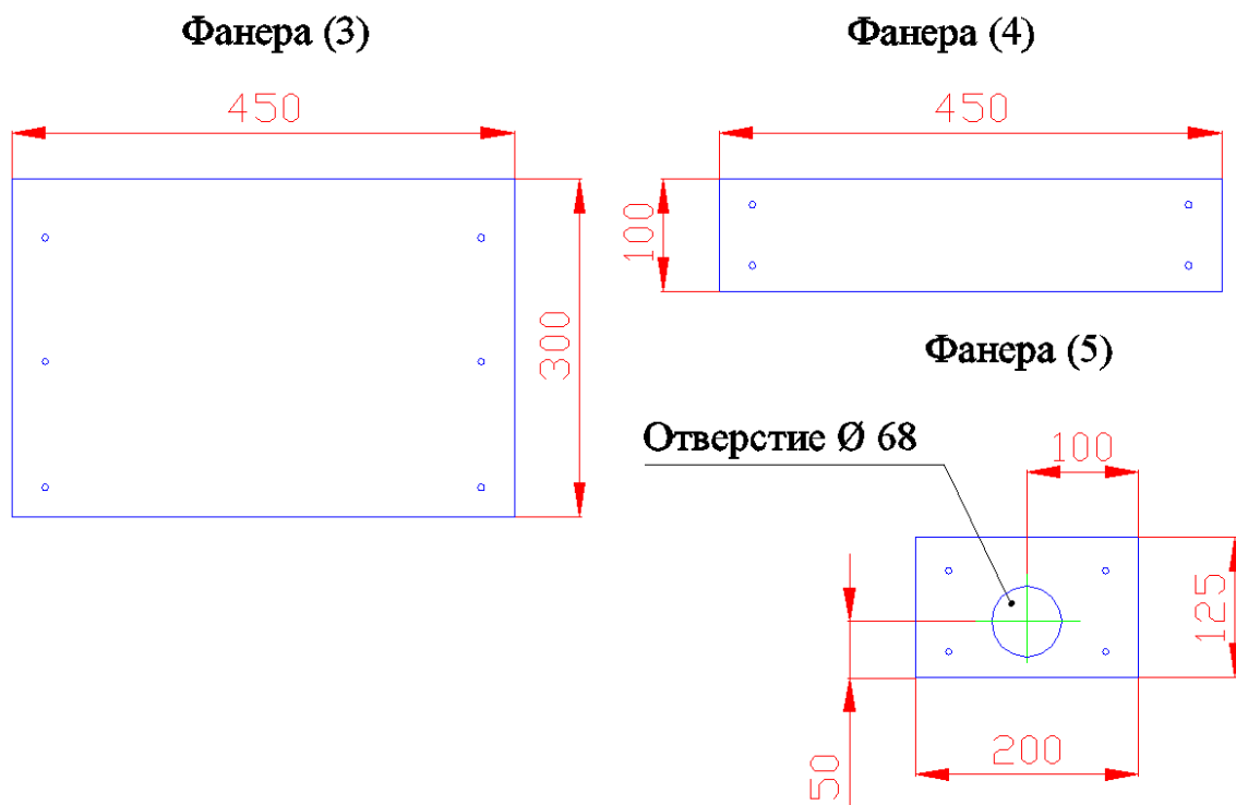
Рисунок 13 (переливной бассейн)
