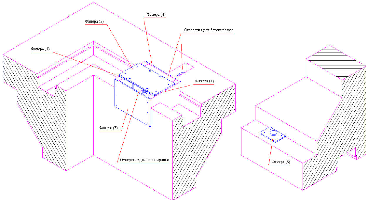
Рисунок 15 (переливной бассейн)
