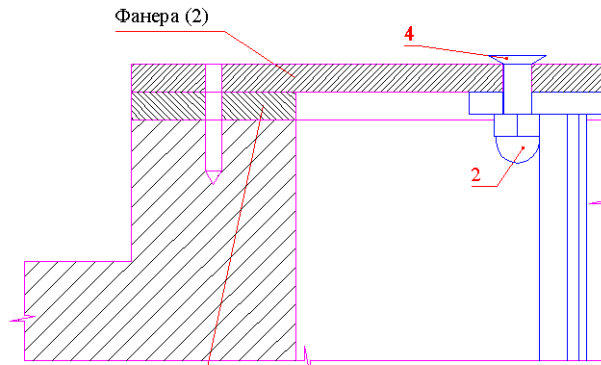
Узел 1
