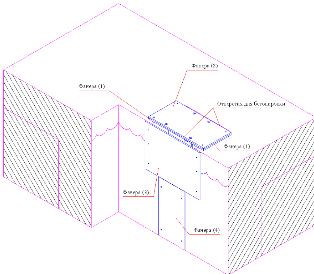
Рисунок 14 (скиммерной бассейн)
