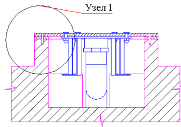
Узел 1
