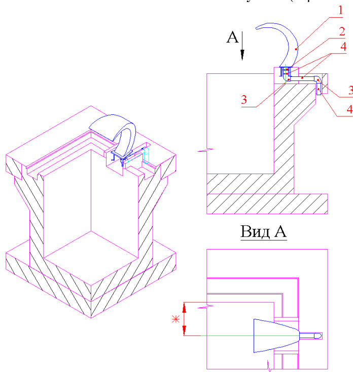
Рисунок 6 (переливной бассейн)
