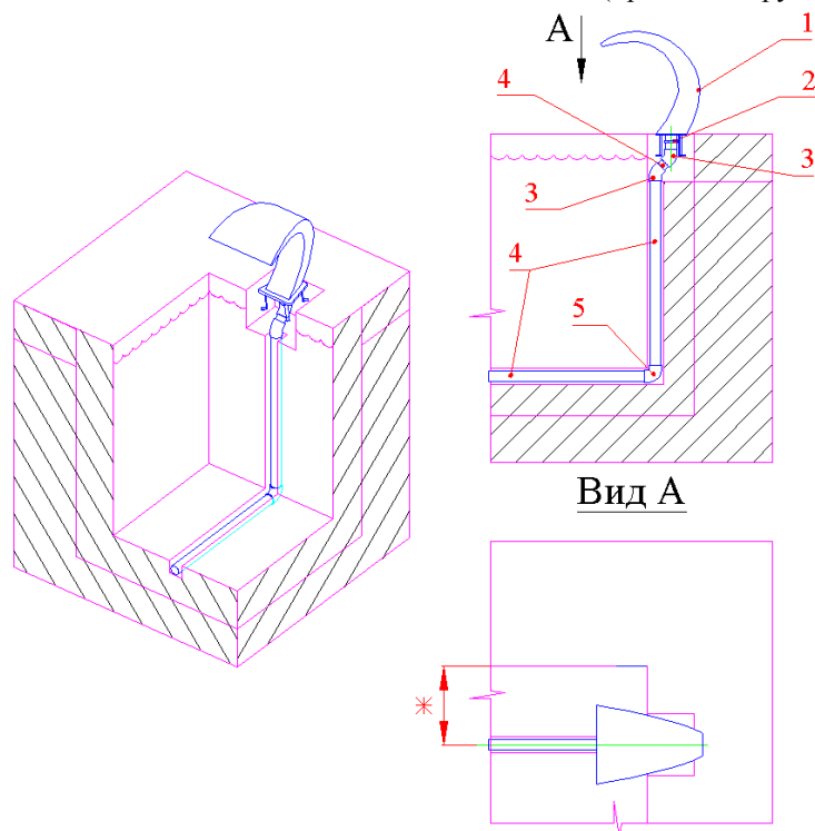
Рисунок 5 (скиммерной бассейн) (прокладка трубопроводов по дну бассейна)
