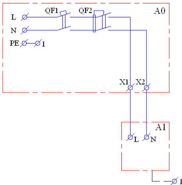
Электрическая схема 1
