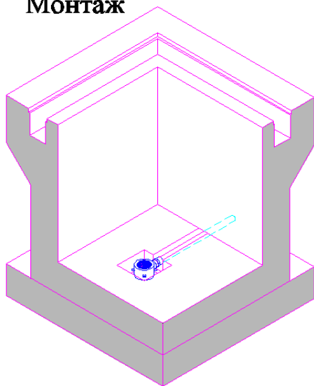
Рисунок 6 (установка слива сквозь борт)
