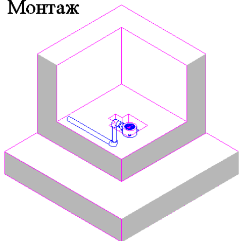
Рисунок 5 (установка слива сквозь дно)
