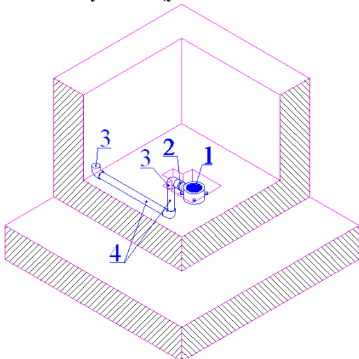
Рисунок 8 (установка сквозь дно)
