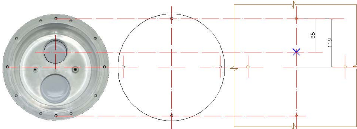
Закладной узел
