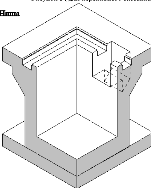
Рисунок 8 ( для переливного бассейна)
