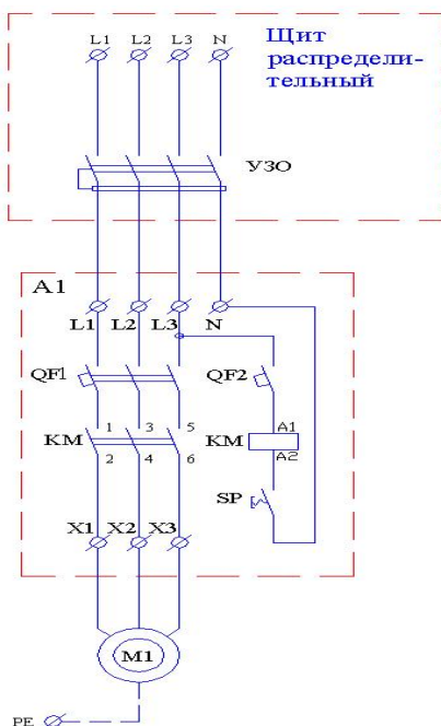
Эл.схема 1
