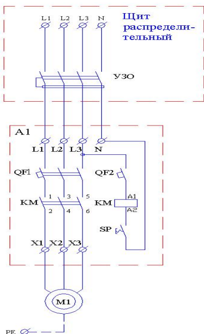
Эл.схема 1
